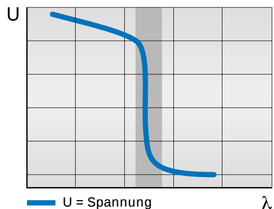
Planar-Lambda-Sonde (Nachkatsonde)
